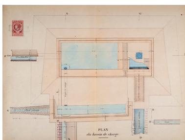
Projet d'exécution des ouvrages hydrauliques et des bâtiments. Dessins de détail du bassin de charge [...], 1903. Phot. Jérôme Mongreville IVR43_20182500161NUC4A
