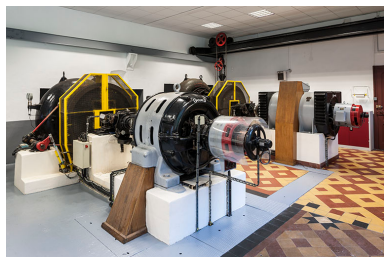
Groupes turbo-alternateurs en service. Phot. Jérôme Mongreville IVR43_20152501772NUC4A
