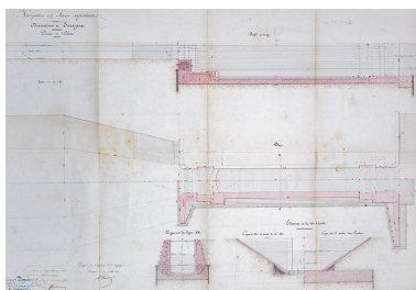
Achèvement du bief de Savoyeux - Allongement et approfondissement de l'écluse à sas de Savoyeux (1882). Phot. Jérôme Mongreville, Autr. Gustave Bouvaist IVR43_20207000116NUC4A
