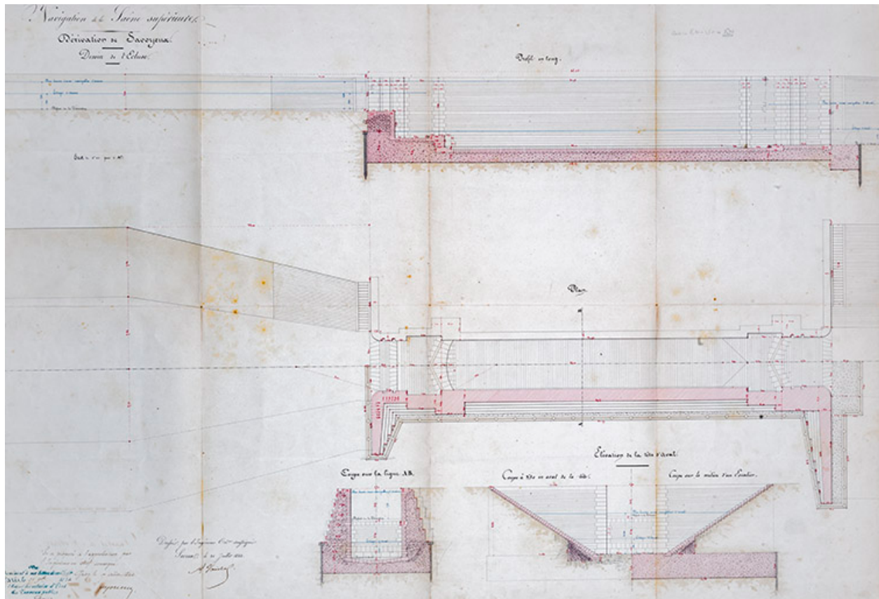
Dérivation de Savoyeux - dessin de l'écluse (1844).
