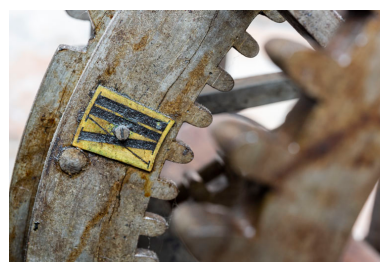
Corps arrière droit (sonnerie des quarts d'heure) : plaque en laiton rivée sur la roue de compte.
