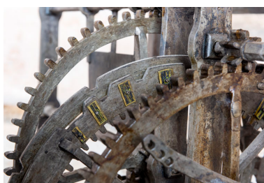
Corps arrière droit (sonnerie des quarts d'heure) : détail de la roue de compte.
