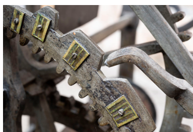
Corps avant gauche (sonnerie des heures) : détail de la roue de compte.
