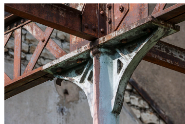
Détail de la charpente métallique. Phot. Jérôme Mongreville IVR43_20142501254NUC4A
