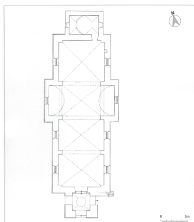
Plan au sol. Dess. Jérôme Mongreville IVR43_20003900825A1
