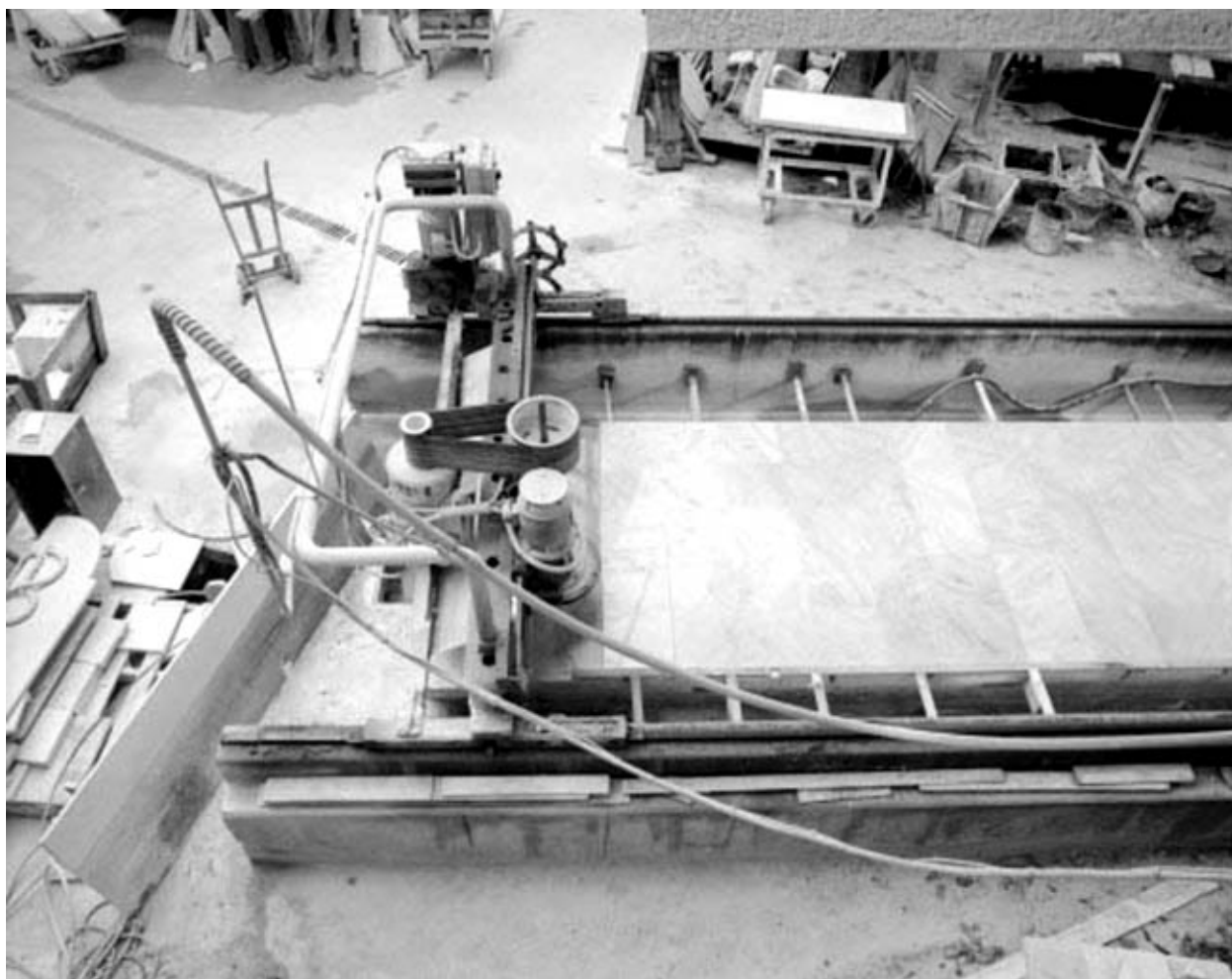
Polissoir ouest : vue plongeante sur le bâti mobile.
