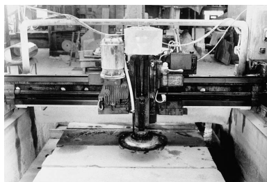
Polissoir est : bâti mobile et plateau de polissage. Phot. Yves Sancey IVR43_19933900487ZA
