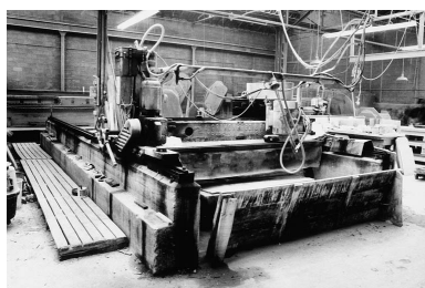
Polissoir est, vu de trois quarts gauche. Phot. Yves Sancey IVR43_19933900486ZA
