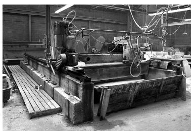
Polissoir est, vu de trois quarts gauche. Phot. Yves Sancey IVR43_19933900339X
