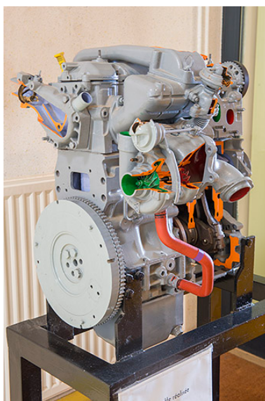
Bloc moteur écorché.
