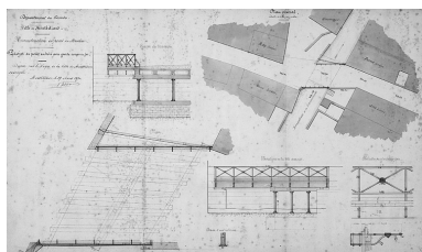
Projet de reconstruction en bois, 1870.
