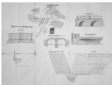
Projet de reconstruction en bois, 1872.
