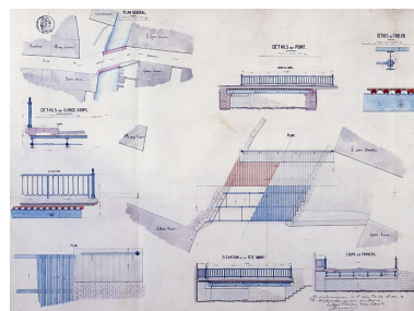
Projet de reconstruction en métal, 1873.
