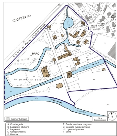
Plan-masse et de situation. Extrait du plan cadastral numérisé, 2008, section A, 1:1250 réduit à 1:2300. Source : Direction générale des Finances Publiques - Cadastre ; mise à jour : 2008. Dess. André Céréza IVR43_20087000343NUDA
