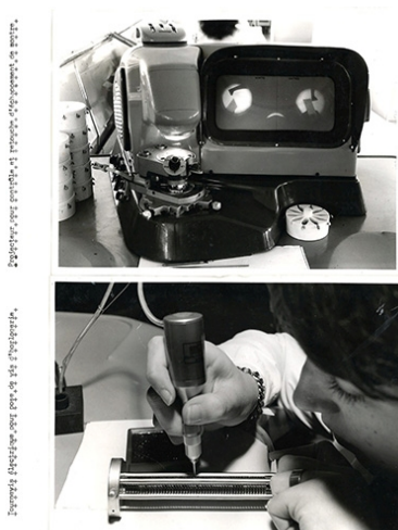
Société Yema : Projecteur pour contrôle et retouche des échappements, et assemblage par vissage électrique, photogr., s.d. [vers 1970]. IVR43_20212500115NUC2A
