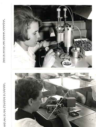
Société Yema : postes de montage (vissage automatique) et de mise en équilibre des balanciers, photogr., s.d. [vers 1970]. IVR43_20212500118NUC2A
