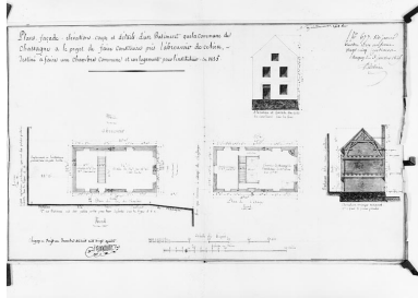
Projet de mairie-école daté 1824 (non réalisé). Dessin aquarellé par Jaquinot J.D. père (architecte). Phot. , Autr. Jaquinot J.D. père (architecte) IVR26_19802101651V
