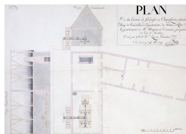
Plan de la tirerie de fil-de-fer et chaufferie [...] appartenant à Mrs Migeon et Dominé [coupe longitudinale, coupe transversale et plan au sol]. Phot. Jérôme Mongreville, Autr. NEPASUTILISERParent (géomètre) IVR43_20019000052VA
