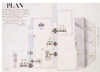
Plan de la tirerie de fil-de-fer, chauffeerie, marteaux à épailler et martinets à filières [...] [coupe longitudinale et plan au sol]. Phot. Jérôme Mongreville, Autr. NEPASUTILISERParent (géomètre) IVR43_20019000042VA
