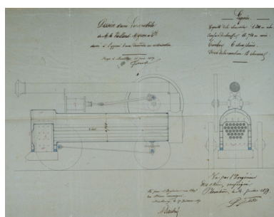
Dessin d'une locomobile de MM. Viellard-Migeon et Cie dressé à l'appui d'une demande en autorisation [coupes longitudinale et transversale]. Phot. Jérôme Mongreville IVR43_20019000230XA
