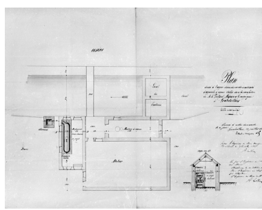
Plan dressé à l'appui d'une demande en autorisation d'appareils à vapeur établis dans la manufacture de MM. Viellard-Migeon et Cie à Grandvillars. Phot. Jérôme Mongreville IVR43_20019000010V
