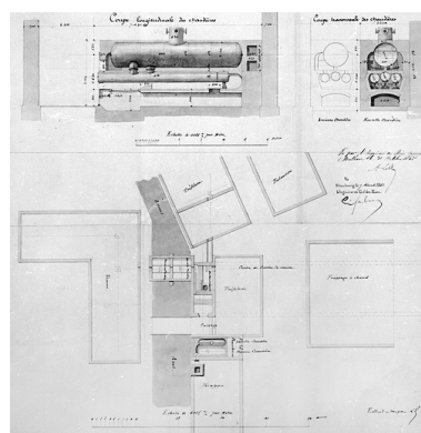
Plan-masse et coupes longitudinale et transversale des chaudières. Phot. Jérôme Mongreville IVR43_20019000005V
