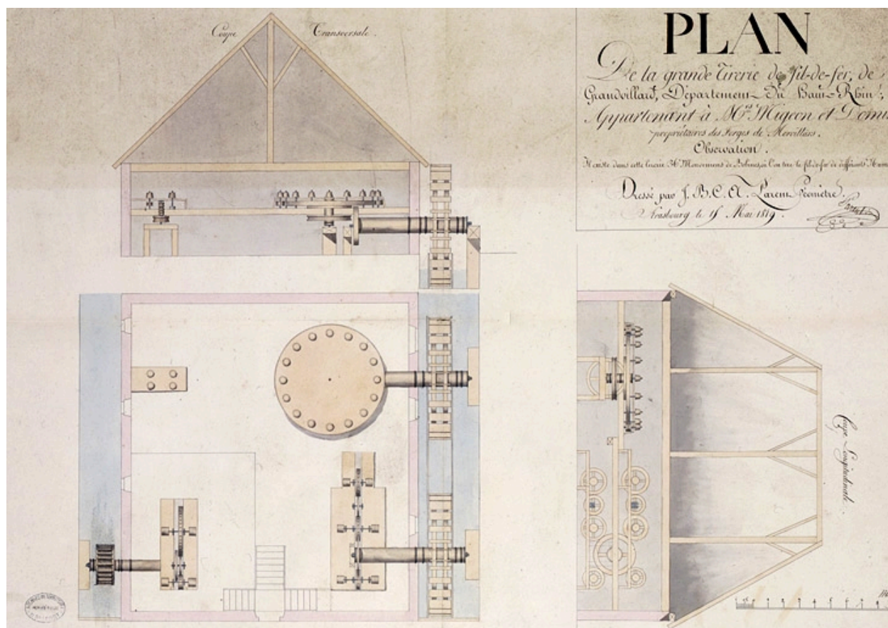
Plan de la grande tirerie de fil-de-fer de Grandvillard [...] [coupe longitudinale, coupe transversale et plan au sol].
