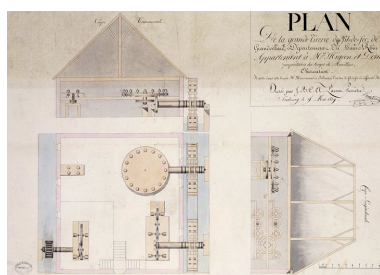
Plan de la grande tirerie de fil-de-fer de Grandvillard [...] [coupe longitudinale, coupe transversale et plan au sol]. Phot. Jérôme Mongreville, Autr. NEPASUTILISERParent (géomètre) IVR43_20019000048VA
