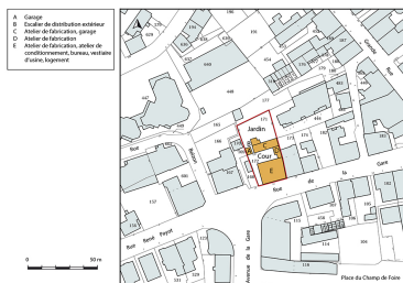
Plan-masse et de situation. Extrait du plan cadastral, 2017, section AA, 1/1 000. Dess. Bertrand Turina IVR43_20182501350NUDA
