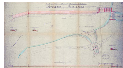
Société Electrique de Belchamp. Station du Châtelot. Déversoir et prise d'eau, pièce n° 6, 1934. Phot. Jérôme Mongreville, Autr. auteur inconnu IVR43_20132500488NUC4A
