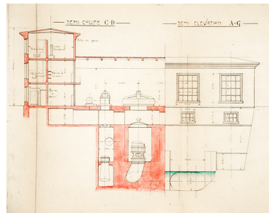
Usine électrique du Châtelot, demi- coupe et demi-élévation, 1917. Phot. Jérôme Mongreville, Autr. auteur inconnu IVR43_20132500495NUC4A
