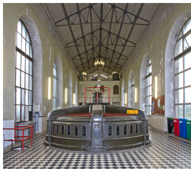
Groupe turbo-alternateur n°1. Phot. Yves Sancey IVR43_20122502051NUC2A
