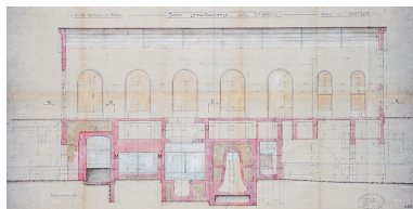
Société Electrique de Belchamp. Station du Châtelot. Coupe longitudinale de l'usine, pièce n° 11, 1934. Phot. Jérôme Mongreville, Autr. auteur inconnu IVR43_20132500485NUC4A
