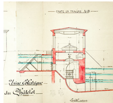
Usine électrique du Châtelot, coupe en travers, 1917. Phot. Jérôme Mongreville, Autr. auteur inconnu IVR43_20132500496NUC4A
