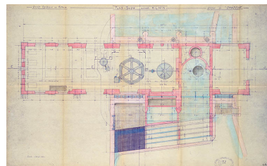
Société Electrique de Belchamp. Station du Châtelot. Plan-coupe de l'usine, pièce n° 9, 1934. Phot. Jérôme Mongreville, Autr. auteur inconnu IVR43_20132500486NUC4A
