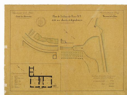
"Plan de l'écluse de Baye n°1 et de ses abords et dépendances".
