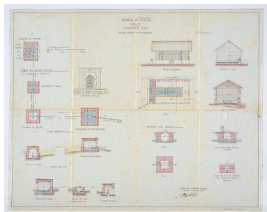
Commune de Corre. Projet d'adduction d'eau. [plans, coupes, élévations.] 1910 Phot.
