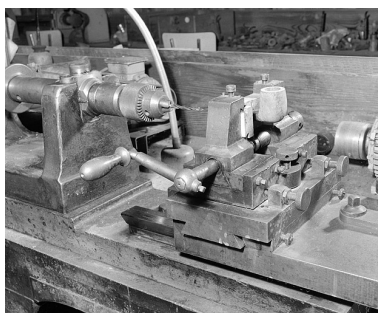
Le chariot mobile et le mandrin porte-mèche, de trois quarts droite (atelier principal). Phot. Jérôme Mongreville IVR43_20022500639X
