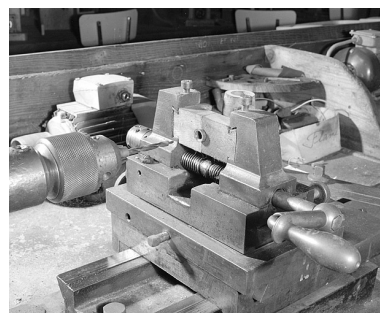
Le chariot mobile et le mandrin porte-mèche, de trois quarts gauche (atelier principal). Phot. Jérôme Mongreville IVR43_20022500640X
