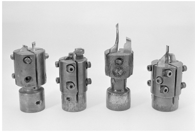
Détail de quatre outils de coupe.
