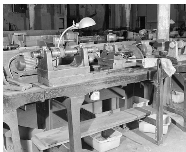
Vue d'ensemble d'une des machines encore munie de sa ceinture (atelier principal). Phot. Jérôme Mongreville IVR43_20022500638X
