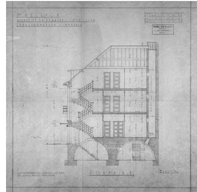
M. Nélaton [...] Transformation d'immeuble. Coupe A.B. (coupe transversale). Phot. Jérôme Mongreville, Autr. Michel-Max (architecte) Claudet IVR43_19893900211X
