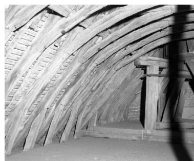
Charpente du comble Phot. Michel Thierry IVR26_19852101218X
