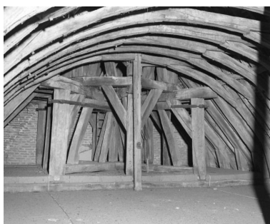
Charpente du comble et beffroi Phot. Michel Thierry IVR26_19852101217X
