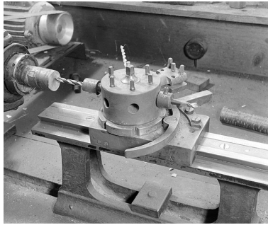
Détail du barillet du tour de gauche (atelier principal). Phot. Jérôme Mongreville IVR43_20022500627X
