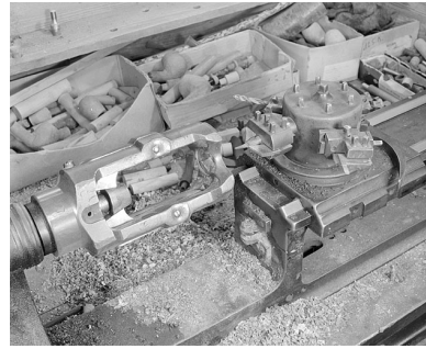
Tour (atelier de finissage). Les mâchoires et le revolver alignés. Phot. Jérôme Mongreville IVR43_20022500476X
