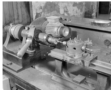
Vue d'ensemble rapprochée du tour de gauche (atelier principal). Phot. Jérôme Mongreville IVR43_20022500628X
