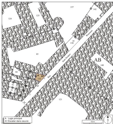
Plan masse et de situation. Extrait du plan cadastral, 1974, section AB. Dess. André Céréza IVR43_20102500023NUDA
