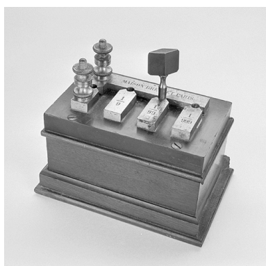
Shunt : vue d'ensemble. Phot. Jérôme Mongreville IVR43_20032500882X
