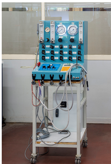
Banc de contrôle pour pièces à main et contres-angle. Phot. Jérôme Mongreville IVR43_20182501258NUC4A
