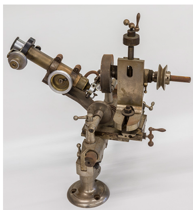
Tailleuses de tire-nerfs. Phot. Jérôme Mongreville
