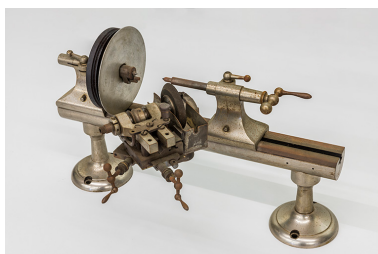
Touret d'affûtage (1957). Phot. Jérôme Mongreville IVR43_20182501259NUC4A
