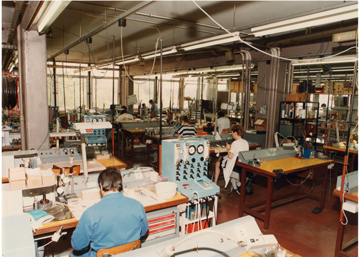
Atelier de montage (contre-angles et pièces à main dentaire), vers 1995.
