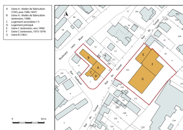
Plan-masse et de situation. Extrait du plan cadastral, 2019. Dess. Bertrand Turina IVR43_20192501110NUDA
