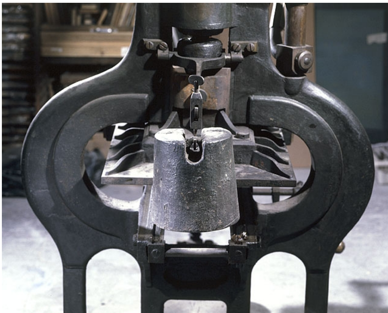
Contrepoids de remontée de la platine.
