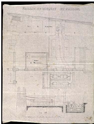
Saline de Melcey et Fallon [plan de la salle des machines]. Phot. Jérôme Mongreville, Phot. Lamare IVR43_20057000560NUCA
