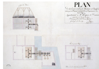
Plan de la tirerie de fil-de-fer, martinet et chaufferie, situés près du Château de Grandvillard [coupe transversale, plan au sol et plan du 1er étage]. Phot. Jérôme Mongreville, Phot. Parent IVR43_20019000038VA
