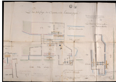
2e feuille de plan des usines de Conflandey [...] Plan et coupe du haut fourneau, plan de la forge, des courants et du laminage projeté. Phot. Daniel Lebée, Autr. Beaujard IVR43_19907000208XA
