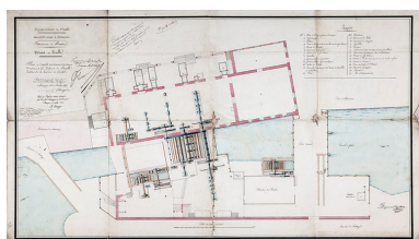
Plan de détails des diverses machines composant les usines de Gouille, 1833. Phot. Jérôme Mongreville IVR43_20152500598NUC4A
