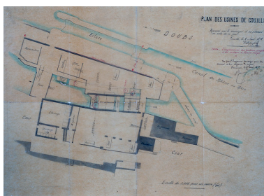
Plan des usines de Gouille, 1872. Phot. Jérôme Mongreville IVR43_20182500088NUC4A
