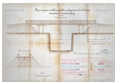
Projet d'un pont à treillis avec palées en charpente sur les écluses des dérivations en dessous de Gray, 1844. Phot. Jérôme Mongreville, Autr. Jean Auguste Philibert Alexandre dit Philippe Lacordaire IVR43_20197000438NUC4A
