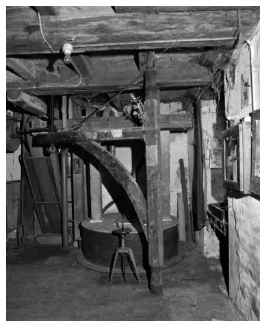
Rez-de-chaussée. Meules, potence et compas. Phot. Jean-Luc Duthu IVR26_20062106672X
