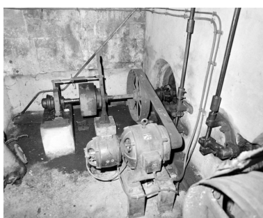
Etage de soubassement. Turbine et générateurs. Phot. Jean-Luc Duthu IVR26_20062106642X
