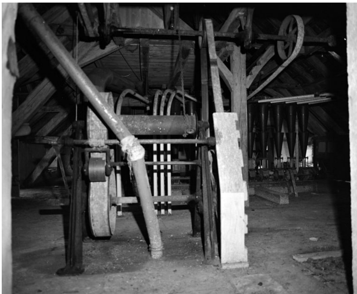
Comble à surcroît. Monte-sacs.
