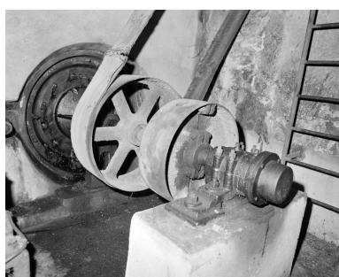
Etage de soubassement. Turbine. Phot. Jean-Luc Duthu IVR26_20062106640X
