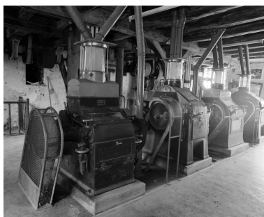
Rez-de-chaussée. Broyeurs (Ateliers de construction Camus frères, ingénieurs, Tonnerre et Socam, Paris). Phot. Jean-Luc Duthu IVR26_20062106654X
