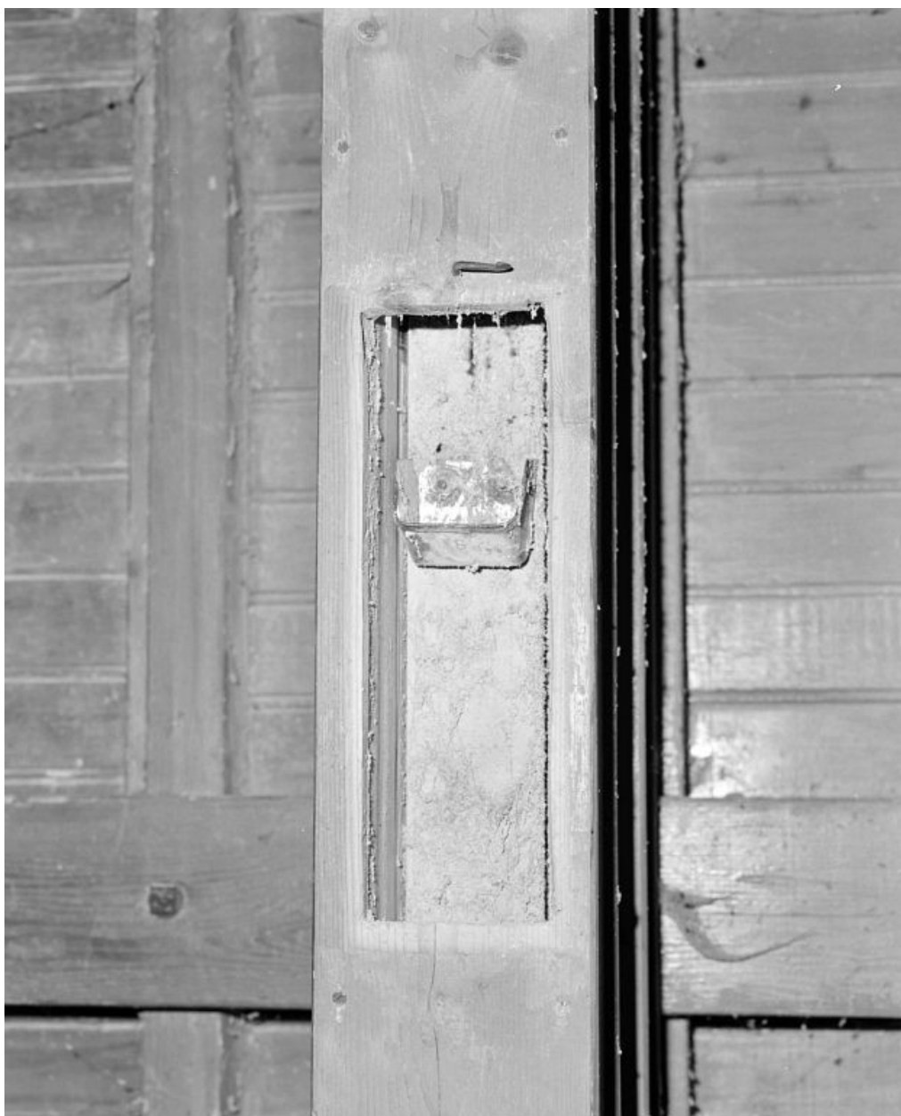
2e étage. Elévateur à godets, détail.
