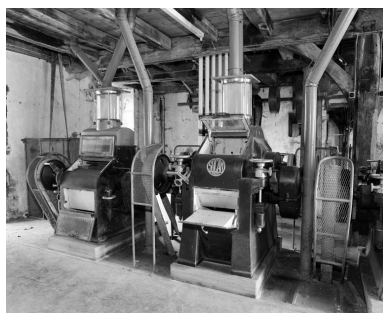
Rez-de-chaussée. Broyeurs (Ateliers de construction Camus frères, ingénieurs, Tonnerre et Socam, Paris). Phot. Jean-Luc Duthu IVR26_20062106658X
