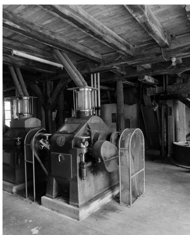
Rez-de-chaussée. Broyeur (marque Socam, Paris). Phot. Jean-Luc Duthu IVR26_20062106648X
