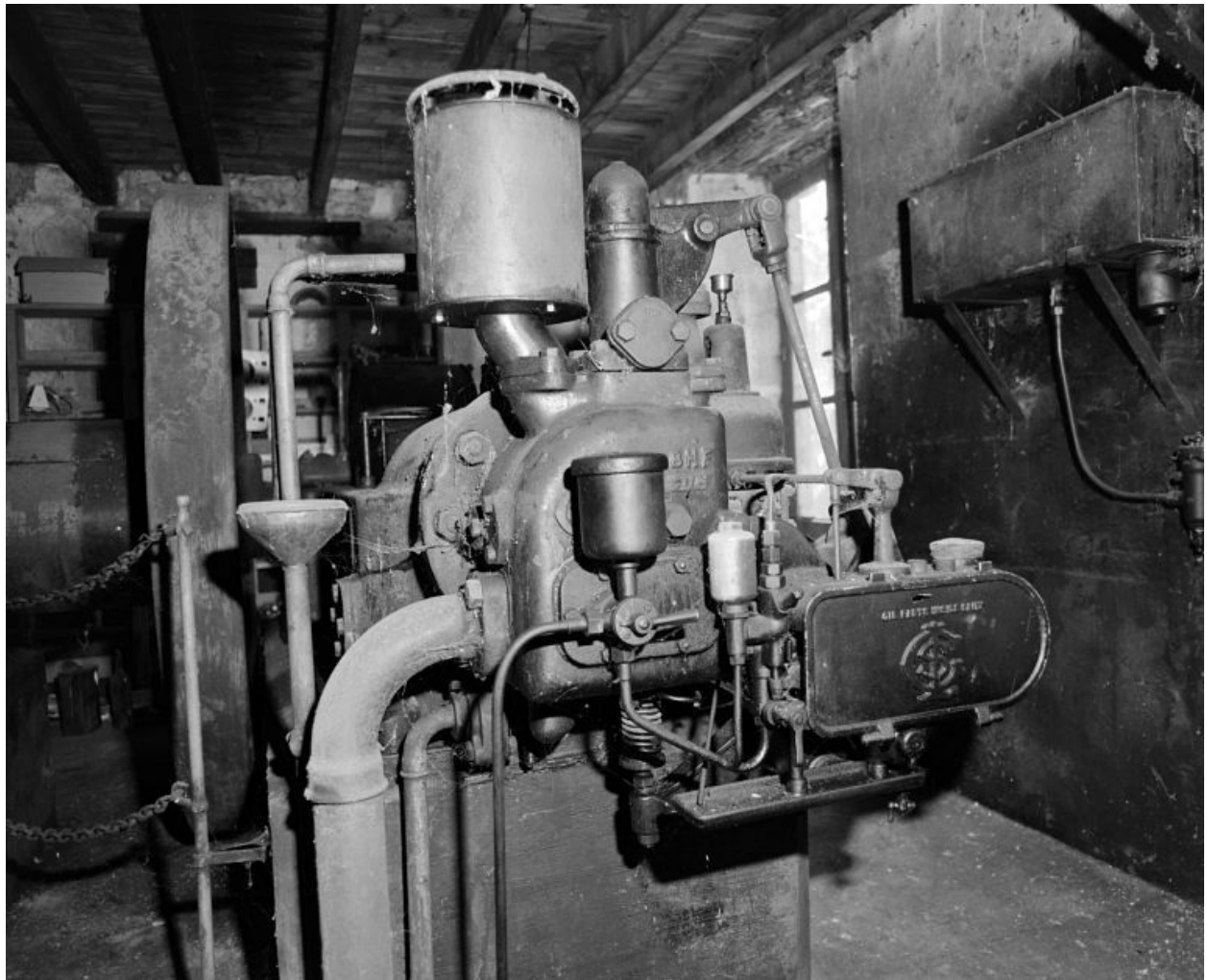
Rez-de-chaussée. Moteur diesel (L. Gardner, constructeur à Patricroft, Angleterre), détail.
