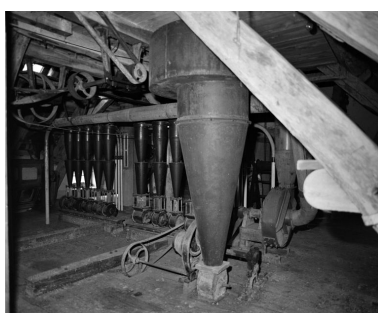
Comble à surcroît. Ecluses. Phot. Jean-Luc Duthu IVR26_20062106744X
