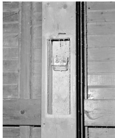
2e étage. Elévateur à godets, détail. Phot. Jean-Luc Duthu IVR26_20062106733X
