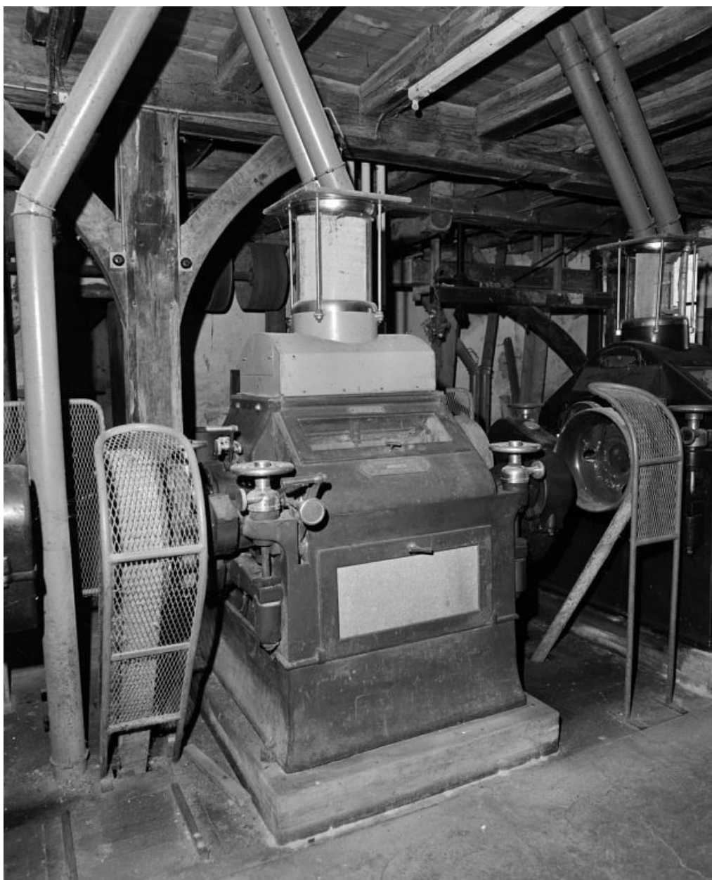
Rez-de-chaussée. Broyeur (marque Buhler et Simon, Uzwil, Suisse).
