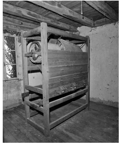
1er étage. Trieur. Phot. Jean-Luc Duthu IVR26_20062106704X
