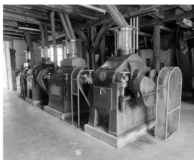
Rez-de-chaussée. Broyeurs. Phot. Jean-Luc Duthu IVR26_20062106646X
