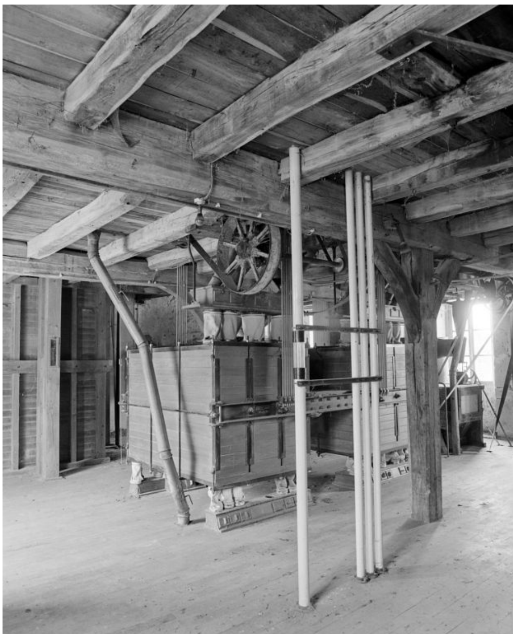
2e étage. Plansichter (Socam, Paris).
