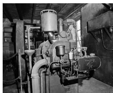
Rez-de-chaussée. Moteur diesel (L. Gardner, constructeur à Patricroft, Angleterre), détail. Phot. Jean-Luc Duthu IVR26_20062106680X
