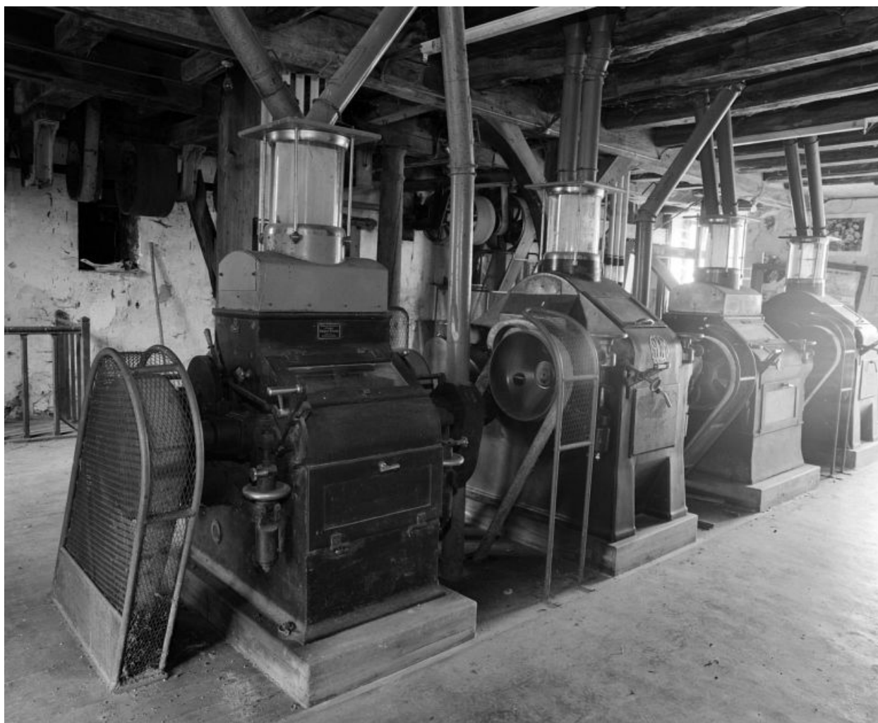
Rez-de-chaussée. Broyeurs (Ateliers de construction Camus frères, ingénieurs, Tonnerre et Socam, Paris).
