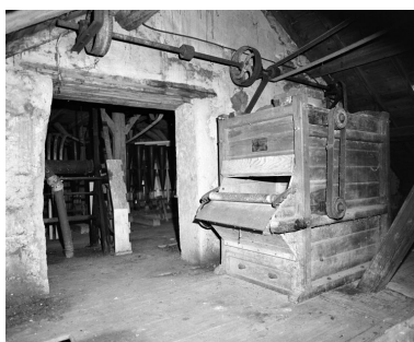
Comble à surcroît. Trieur (anciens établissements Lhuillier, Dijon). Phot. Jean-Luc Duthu IVR26_20062106750X
