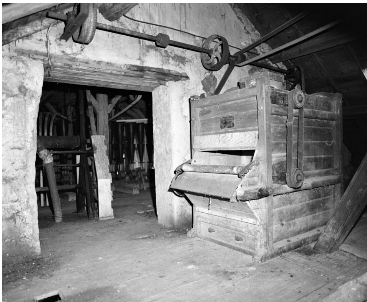
Comble à surcroît. Trieur (anciens établissements Lhuillier, Dijon).
