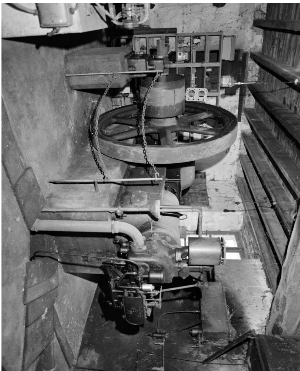
Rez-de-chaussée. Moteur diesel (L. Gardner, constructeur à Patricroft, Angleterre).
