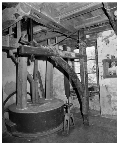
Rez-de-chaussée. Meules, potence et compas. Phot. Jean-Luc Duthu IVR26_20062106670X
