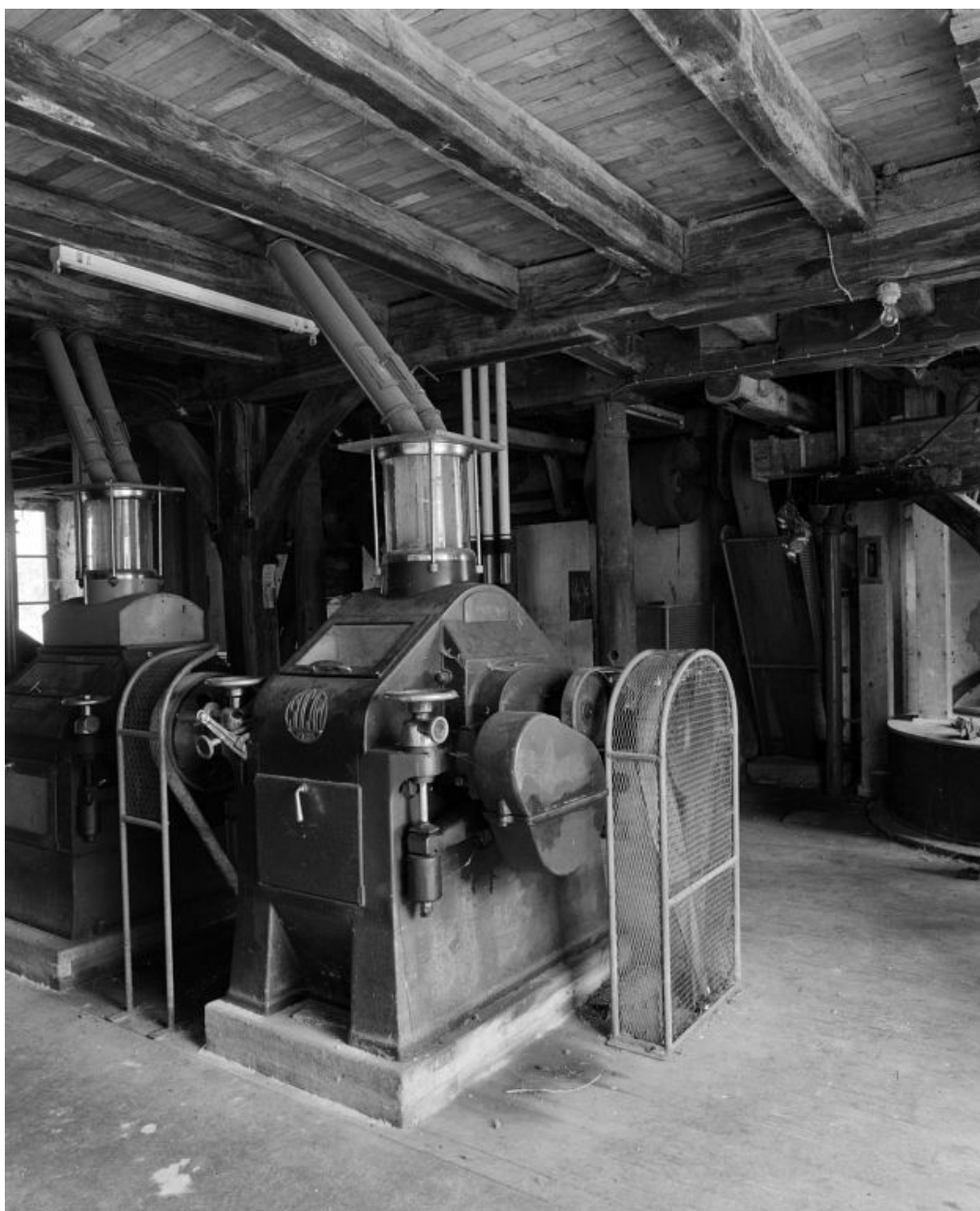
Rez-de-chaussée. Broyeur (marque Socam, Paris).
