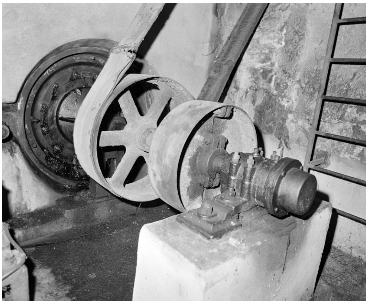
Etage de soubassement. Turbine.
