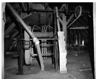
Comble à surcroît. Monte-sacs. Phot. Jean-Luc Duthu IVR26_20062106754X
