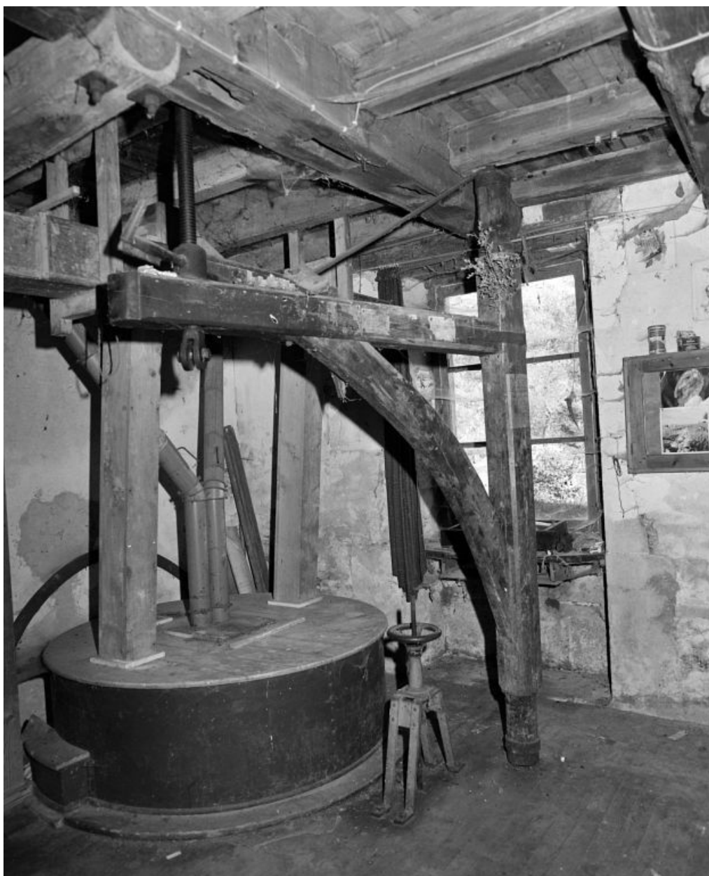
Rez-de-chaussée. Meules, potence et compas.
