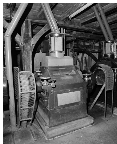
Rez-de-chaussée. Broyeur (marque Buhler et Simon, Uzwil, Suisse). Phot. Jean-Luc Duthu IVR26_20062106650X
