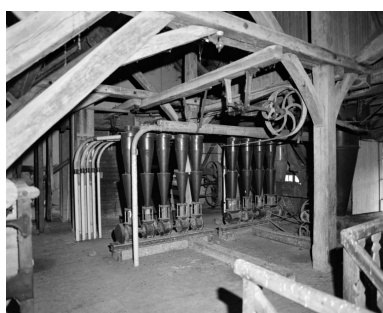
Comble à surcroît. Ecluses. Phot. Jean-Luc Duthu IVR26_20062106742X
