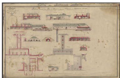
Batterie annexe du Fort d'Asnières - Caserne et bâtiments d'entrée. 1882 [signé par le chef du Génie le 20 avril 1885].
