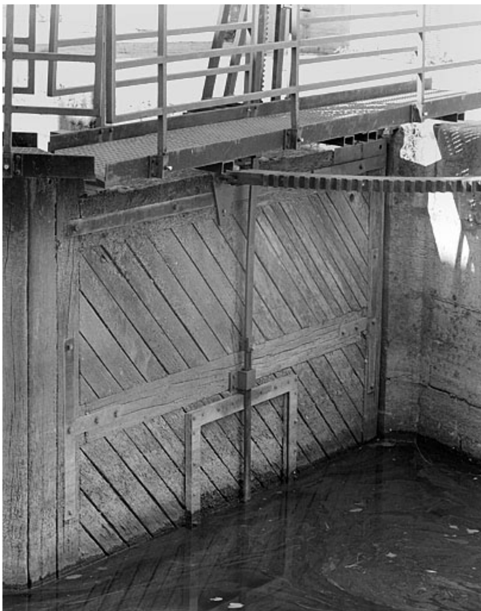
Porte amont droite : tige de manoeuvre et guide de la vantelle.
