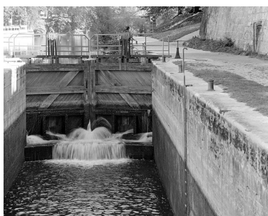
Porte amont droite, face aval. Phot. Jérôme Mongreville IVR43_20032500207X
