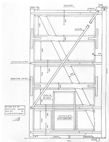
Ecluse n° 50. Porte aval gauche. Vue de la face amont, 1987. Phot. Yves Sancey, Autr. Jacques Avocat IVR43_20062500418NUCA
