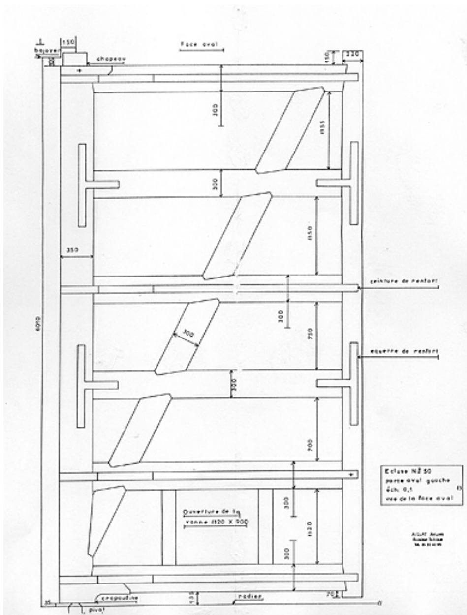
Ecluse n° 50. Porte aval gauche. Vue de la face aval, 1987.
