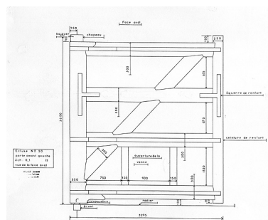
Ecluse n° 50. Porte amont gauche. Vue de la face aval, 1987. Phot. Yves Sancey, Autr. Jacques Avocat
