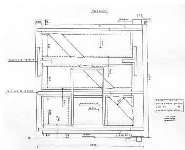
Ecluse n° 50. Porte amont gauche. Vue de la face amont, 1987. Phot. Yves Sancey, Autr. Jacques Avocat
