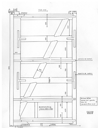
Ecluse n° 50. Porte aval gauche. Vue de la face aval, 1987. Phot. Yves Sancey, Autr. Jacques Avocat IVR43_20062500417NUCA
