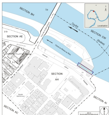
Plan-masse et de situation.
