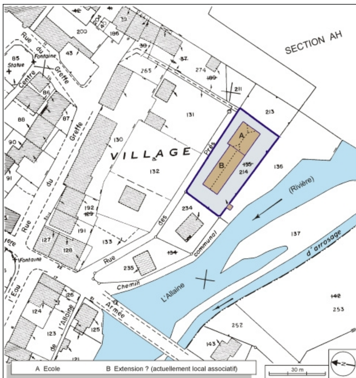
Plan-masse et de situation. Extrait du plan cadastral, 1984, section AI, 1:1000.
