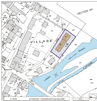
Plan-masse et de situation. Extrait du plan cadastral, 1984, section AI, 1:1000. Dess. André Céréza IVR43_20039000049NUDA
