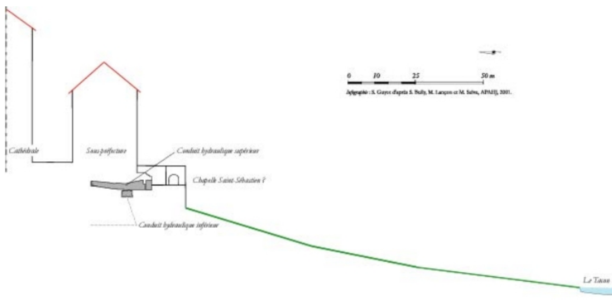
Croquis du conduit hydraulique souterrain.
