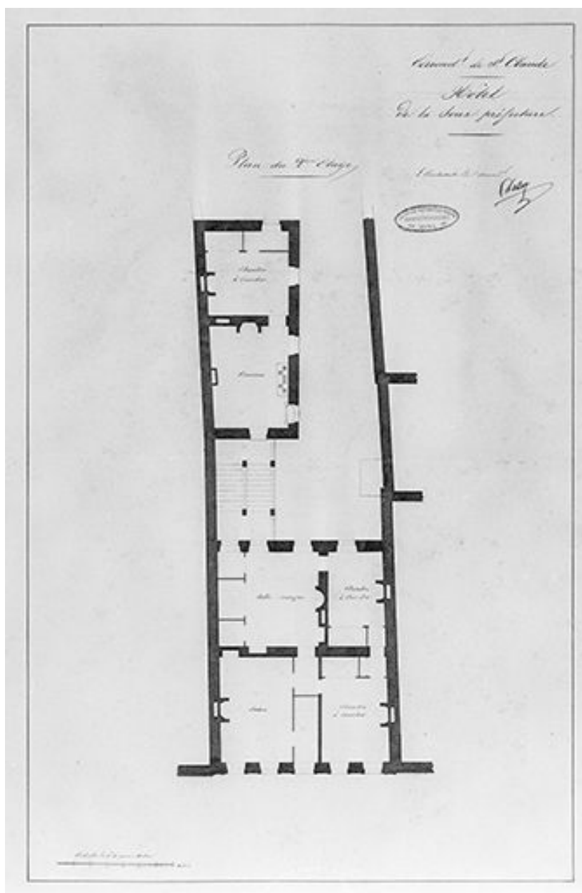
Plan du deuxième étage par Joseph-Marie Dalloz, architecte de la ville, s.d. [19e siècle].
