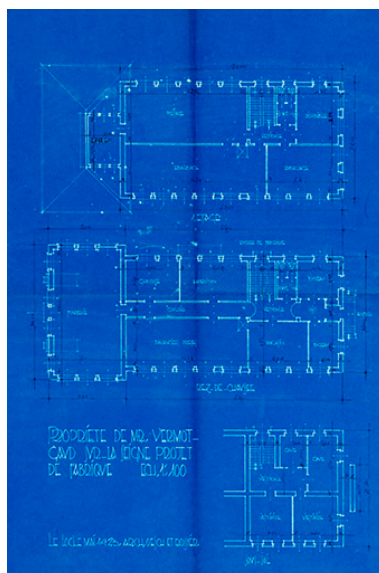
Propriété de Mr Vermot-Gaud, Sur-la-Seigne. Projet de fabrique. Sous-sol, Rez-de-chaussée [et] 1er étage [plans], mai 1923. Phot. Jérôme Mongreville, Autr. Oesch et Rossier
