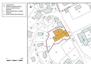
Plan-masse et de situation. Extrait du plan cadastral, 2016, section AB, 1/1 000. Dess. Bertrand Turina IVR43_20182501328NUDA
