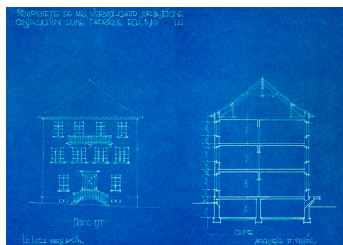
Propriété de Mr Vermot-Gaud, Sur-la-Seigne. Projet de fabrique. Façade est [et] Coupe, mars 1924.
