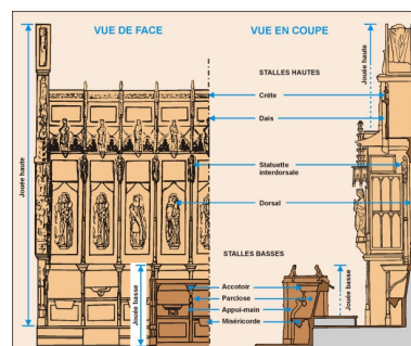
Coupe et élévation des stalles. Dess. André Céréza IVR43_20033900053NUDA
