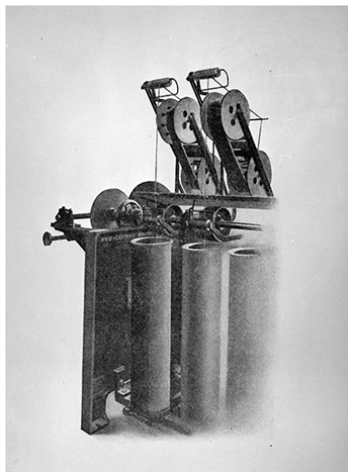
Dévideuse à pots tournants type D.S.P. Phot. Yves Sancey IVR43_19953900126X
