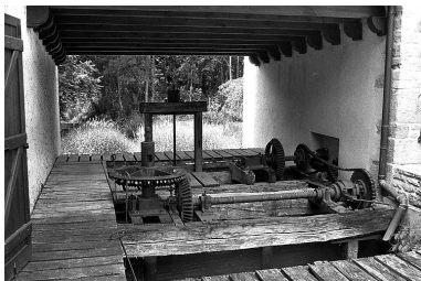
Systèmes d'admission d'eau et de transmission de la turbine. Phot. Laurent Poupard IVR43_19883900562Z
