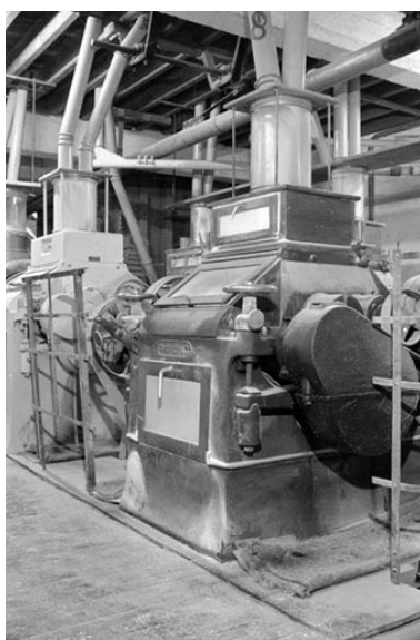
Minoterie, intérieur : appareil à cylindres Buhler. Phot. Laurent Poupard
