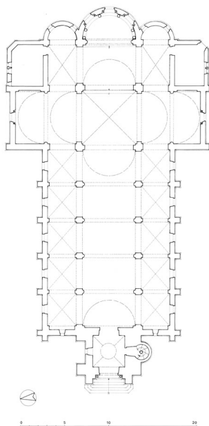
Plan au sol avec indication des couvertures.
