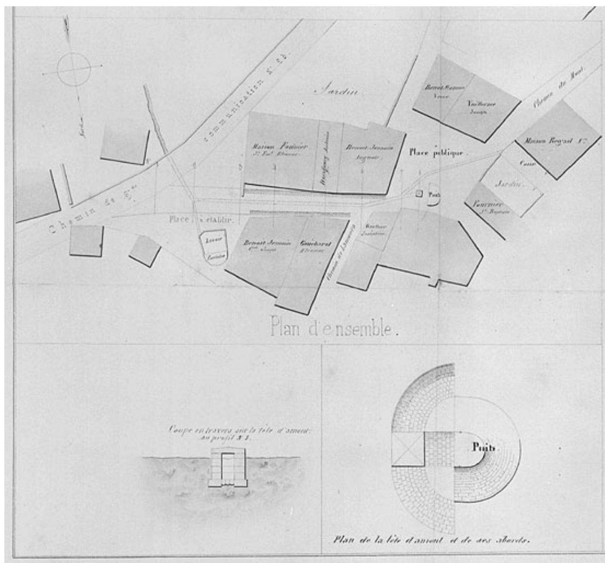
Plan d'ensemble.
