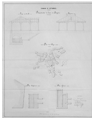
Commune de Septmoncel. Reconstruction du lavoir du Bugnon [plan du village, plan, coupe et façade]. Phot. Jérôme Mongreville, Phot. Auguste Comoy IVR43_19963901864X
