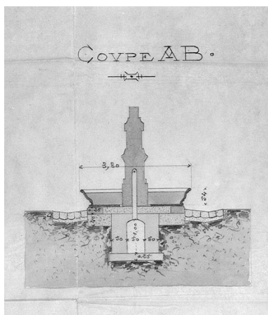
Coupe. Phot. Jérôme Mongreville, Phot. Emile Hytier IVR43_19963901861X
