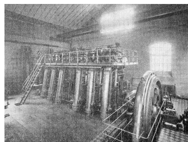
Usine Diesel de Saint-Claude [vue du moteur diesel Carels], en 1935. Phot. Yves Sancey IVR43_19933900128X
