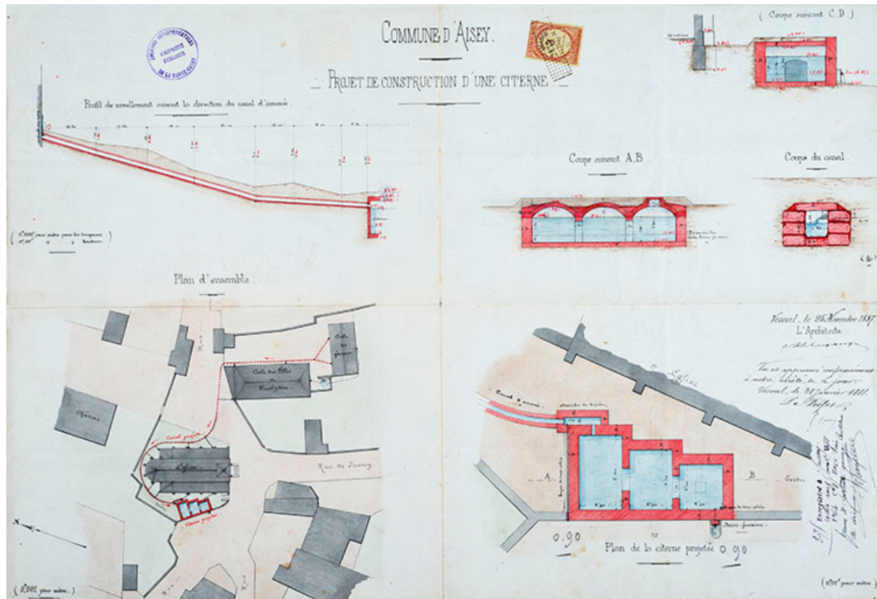
Aménagement d'une citerne à Aisey (1887).
