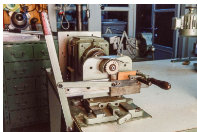
Détail de la fraise (côté fraiseuse). Phot. Jérôme Mongreville IVR43_20003901122ZA
