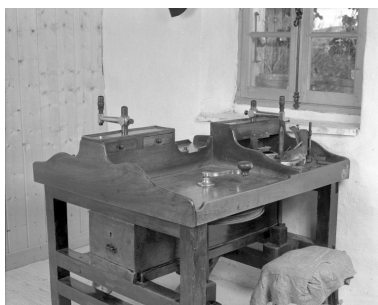
Le plateau et ses 2 postes de travail. Système moteur au premier plan. Phot. Jérôme Mongreville IVR43_19943900722X
