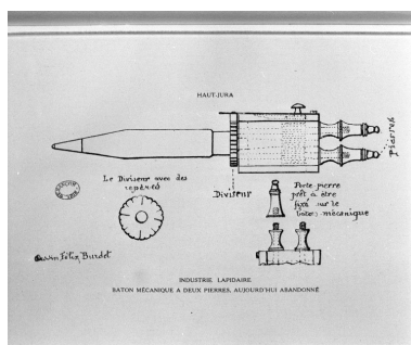
Bâton mécanique à deux pierres, aujourd'hui abandonné. Phot. Jérôme Mongreville, Autr. Félix Burdet IVR43_19943901305X
