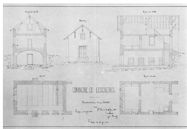
Commune de Leschères, construction d'un chalet [plans, coupes et élévation]. Phot. Jérôme Mongreville, Phot. Auguste Comoy IVR43_19963901751X
