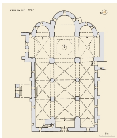
Plan au sol. Dess. André Céréza IVR43_20023900070NUDA
