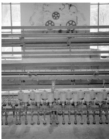
Détail du module de gauche, montrant 15 broches. De bas en haut, système de freinage des broches au pied, broches, système de guidage des fils et moulins. Phot. Yves Sancey IVR43_19943901497X
