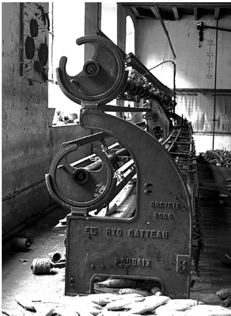
Extrémité gauche de la machine.
