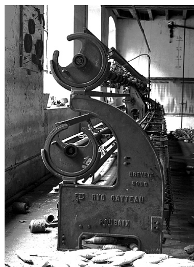
Extrémité gauche de la machine. Phot. Yves Sancey IVR43_19943901495X
