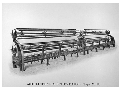
La Moulineuse à écheveaux type MUS. Phot. Yves Sancey IVR43_19953900120X
