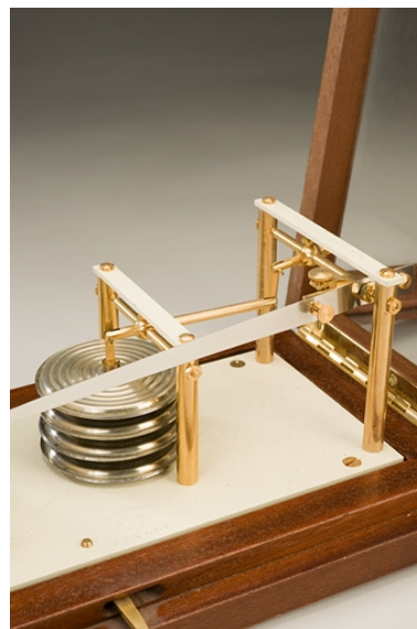
Capsules de Vidié et système de transmission du mouvement à l'aiguille. Phot. Marc Loukachine IVR43_20122500059NUC4A
