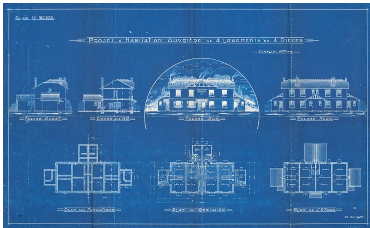
Projet d'habitation ouvrière de 4 logements de 4 pièces.
