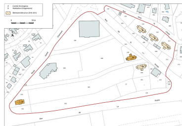
Plan-masse et de situation. Dess. Mathias Papigny IVR43_20132502700NUDA
