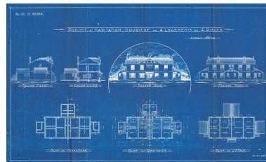
Projet d'habitation ouvrière de 4 logements de 4 pièces. Phot. Jérôme Mongreville, Autr. Eugène (architecte) NEPASUTILISERReess IVR43_20122501173NUC4A
